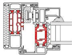
► 58BWST HI OPEN OUT LOCK JAMB
