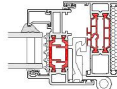
► 58BWST HI OPEN OUT HINGE JAMB
